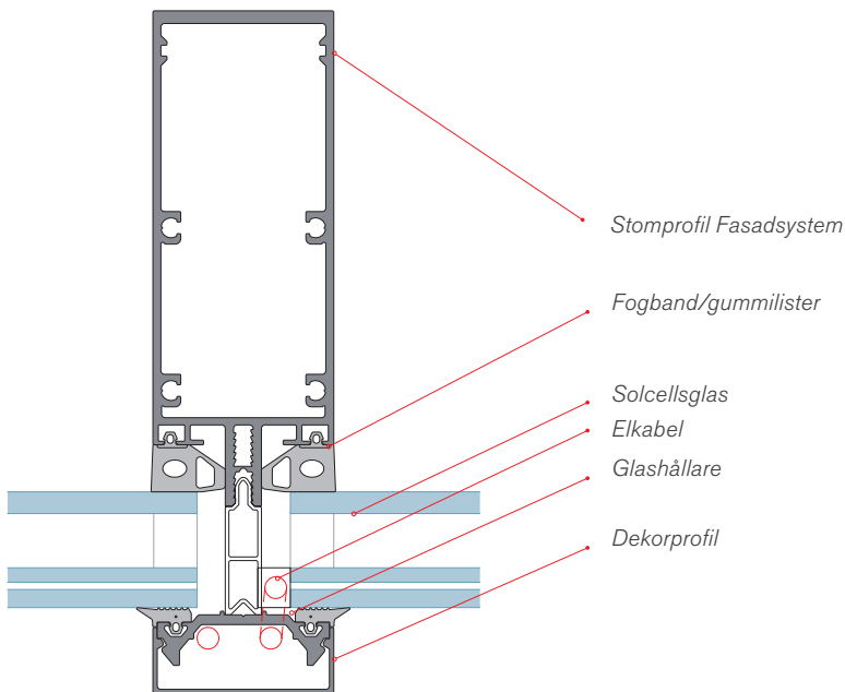
Exempel på integration i fasadsystem. Vertikal stomprofil fasad 4150.
