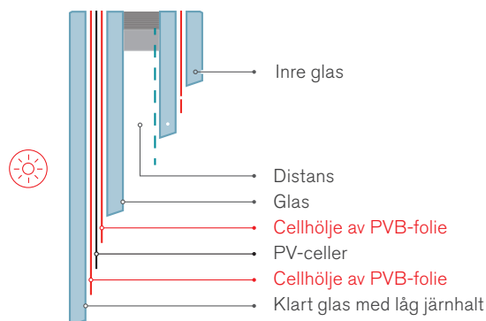
Exempel solcellsglas, uppbyggnad: tvåglas isolerruta, genomsiktigt
