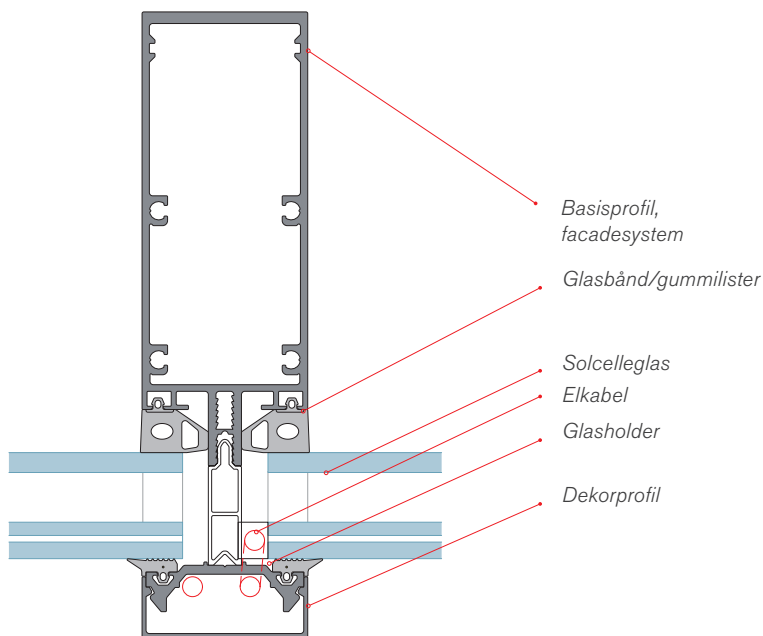
Eksempel på integration i facadesystem. Vertikalt basisprofil, Facade 4150.
