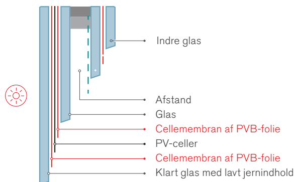
Eksempel på solcelleglassets opbygning (2-lags termorude, gennemsigtig)
