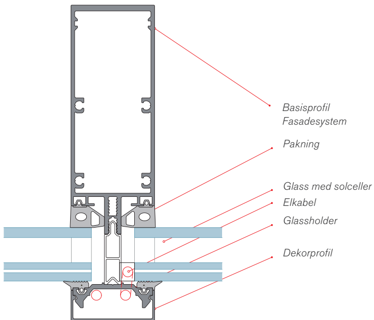
Eksempel på integrering i fasadesystem. Vertikal basisprofil fasade 4150.
