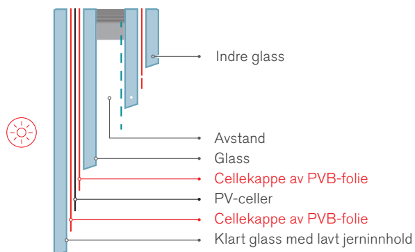
Eksempel på oppbygningen til glass med solceller (2-lags isolerglass, gjennomsiktig)
